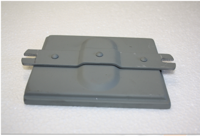
Cover for battery box 4401-18 1918 - 24 Art.no: 4401-18C
